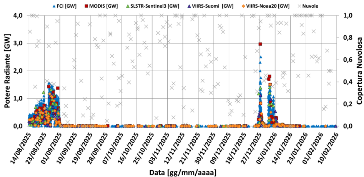
Fig. 8.1 Potere radiante calcolato da dati MODIS (quadrato rosso), SENTINEL-3 SLSTR (triangolo verde), VIIRS (triangolo viola e rombo giallo) e FCI (triangolo blu) dal 14 agosto 2025 al 10 febbraio 2026.
