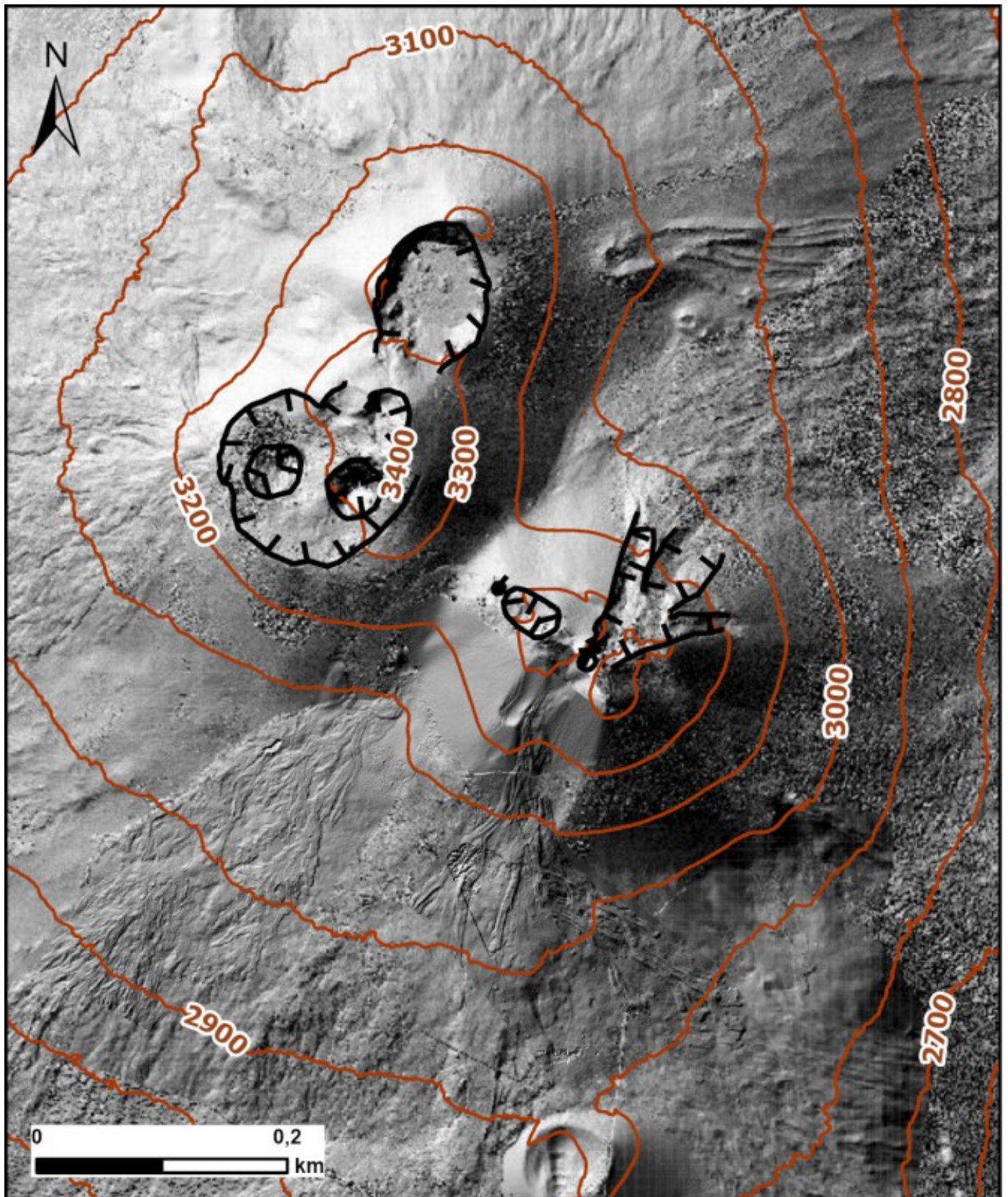
Fig. 3.1 Rilievo ombreggiato dell'area sommitale dell'Etna, ottenuto dall'elaborazione delle immagini acquisite da drone a giugno e ottobre 2025. Le curve di livello geoidiche sono tracciate ogni 100 metri. CSE= cratere di Sud Est, CNE=cratere di Nord Est VOR= Voragine, BN= Bocca Nuova.
