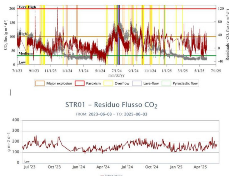
Fig. 6.5 Andamento del flusso medio giornaliero di CO 2 dal suolo negli ultimi due anni misurato a Mofete (sopra) ed a Scari (sotto). Il segnale in rosso nel grafico di Mofete rappresenta il residuo, dopo la correzione per gli effetti delle variabili ambientali.
