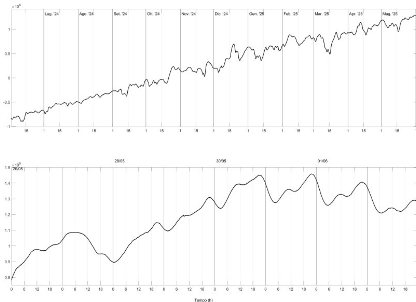
Fig. 4.3 Grafico relativo al dato dilatometrico registrato a SVO: in alto viene mostrato lo strain registrato nell'ultimo anno dal 02/06/2024; in basso quello registrato nell'ultima settimana.
