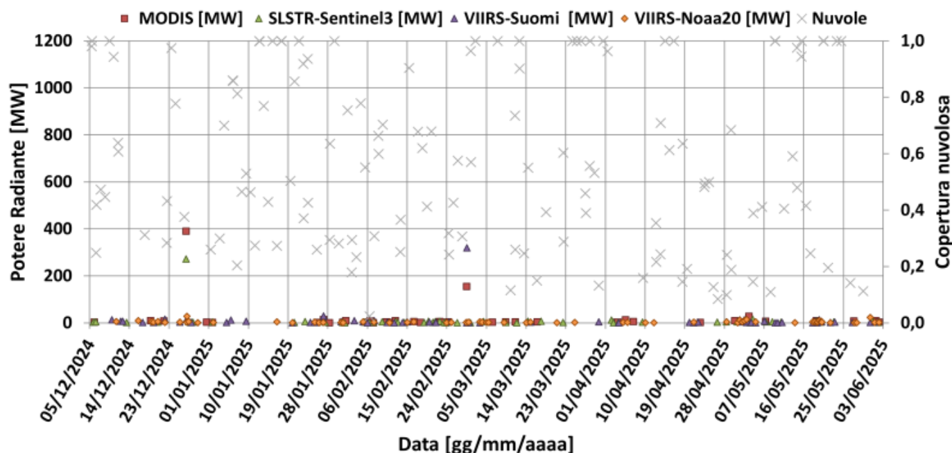
Fig. 7.1 Potere radiante calcolato da dati MODIS (quadrato rosso), SENTINEL-3 SLSTR (triangolo verde) e VIIRS (triangolo viola e rombo giallo) dal 5 dicembre 2024 al 2 giugno 2025.
