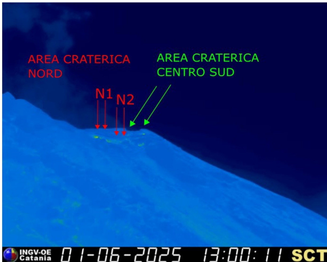
Fig. 3.1 La terrazza craterica vista dalla telecamera termica posta a quota 190 con la delimitazione delle aree crateriche Area Centro-Sud e Area Nord (rispettivamente AREA C-S, AREA N). Le frecce indicano le ubicazioni delle bocche attive.
