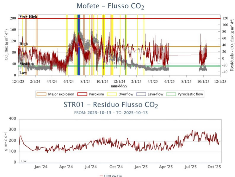
Fig. 6.5 Andamento del flusso medio giornaliero di CO 2 dal suolo registrato a Mofete (sopra) ed a Scari (sotto) negli ultimi due anni.
