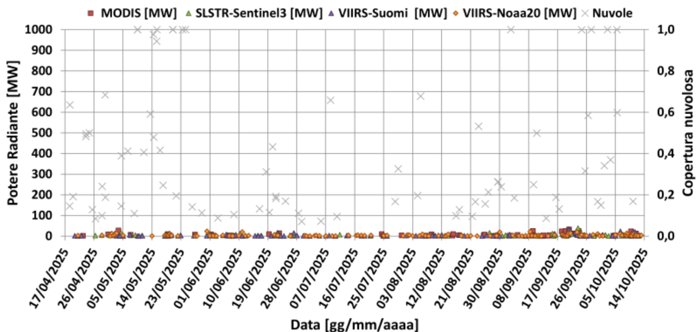
Fig. 7.1 Potere radiante calcolato da dati MODIS (quadrato rosso), SENTINEL-3 SLSTR (triangolo verde) e VIIRS (triangolo viola e rombo giallo) dal 17 aprile 2025 al 14 ottobre 2025.
