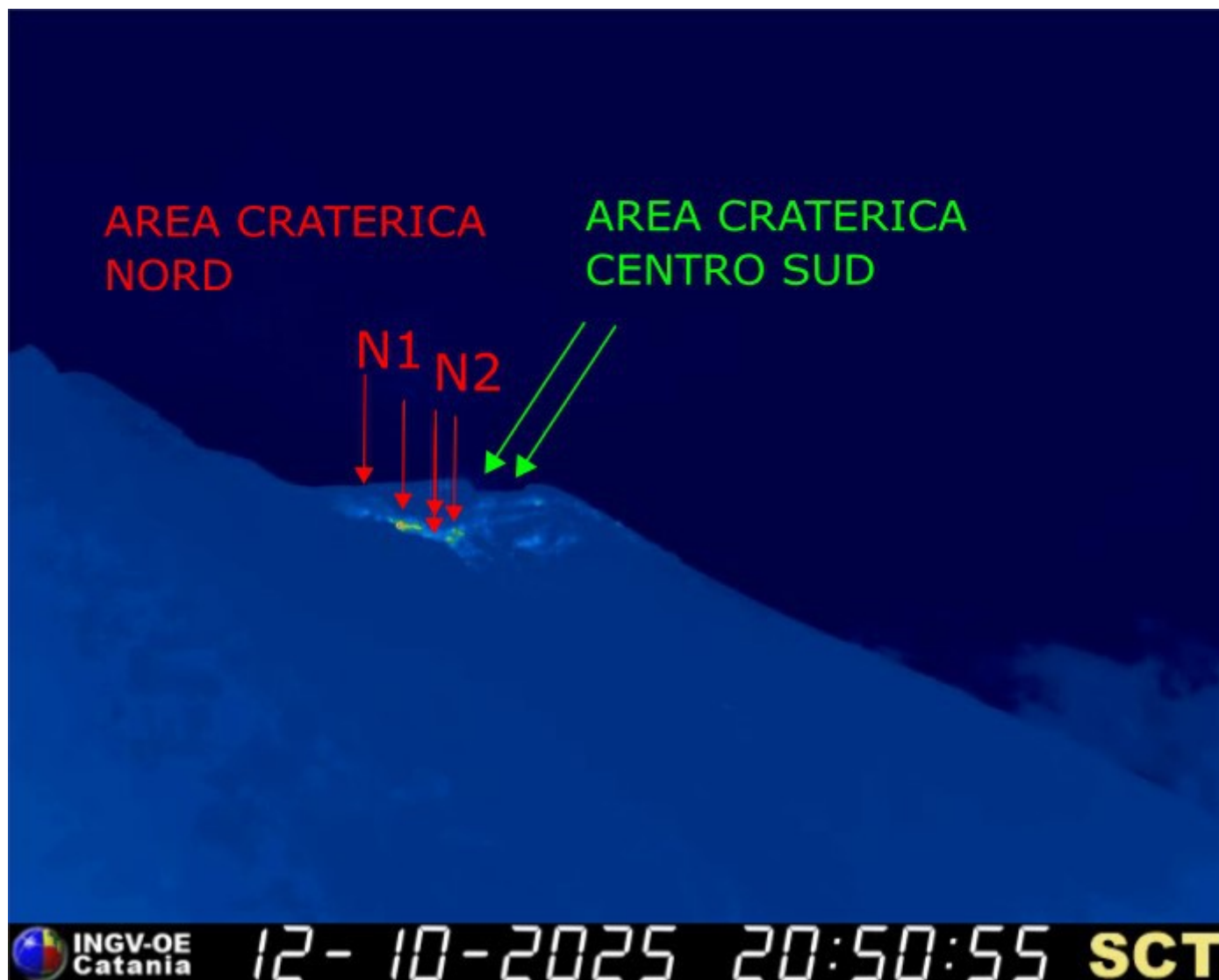
Fig. 3.1 La terrazza craterica vista dalla telecamera termica posta a quota 190, le frecce indicano le bocche attive e le rispettive aree crateriche.
