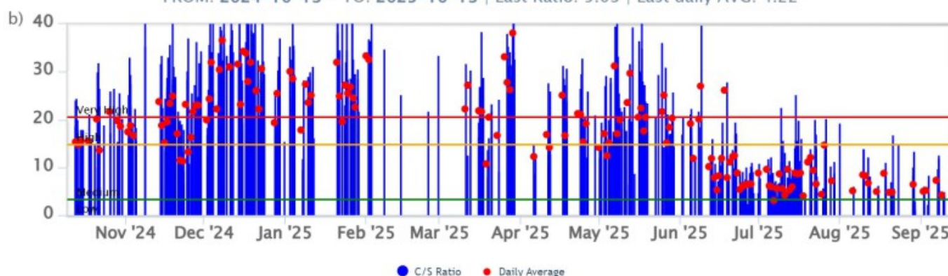
Fig. 6.3 Andamento medio settimanale del rapporto CO_2/SO_2 nel plume: a) Luglio-Settembre; b) ultimo anno.
