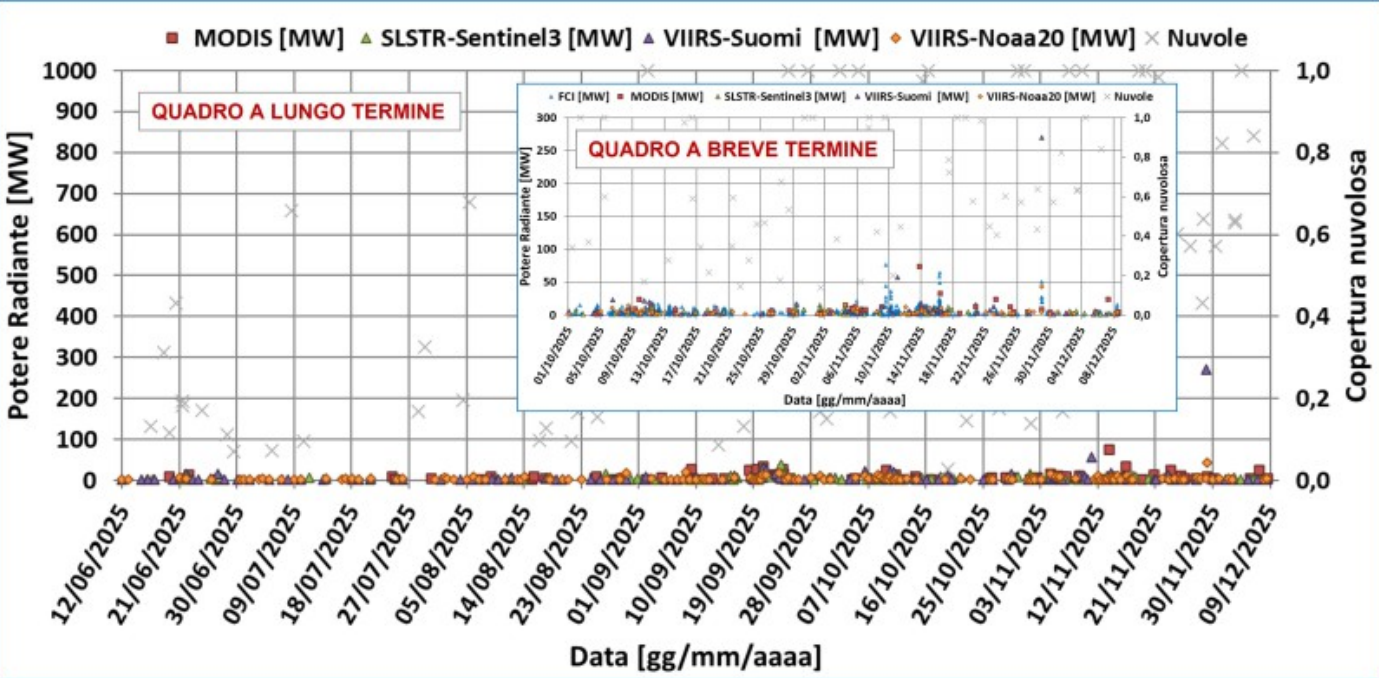
Fig. 7.1 Potere radiante calcolato da dati MODIS (quadrato rosso), SENTINEL-3 SLSTR (triangolo verde), VIIRS (triangolo viola e rombo giallo) e MTG-FCI (triangolo blu) dal 12 giugno 2025 al 9 dicembre 2025.
