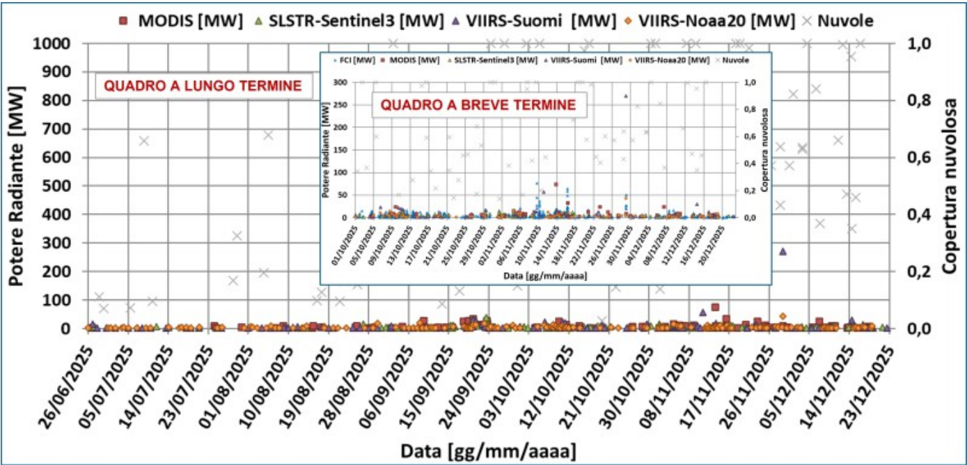
Fig. 7.1 Potere radiante calcolato da dati MODIS (quadrato rosso), SENTINEL-3 SLSTR (triangolo verde), VIIRS (triangolo viola e rombo giallo) e MTG-FCI (triangolo blu) dal 26 giugno 2025 al 23 dicembre 2025.
