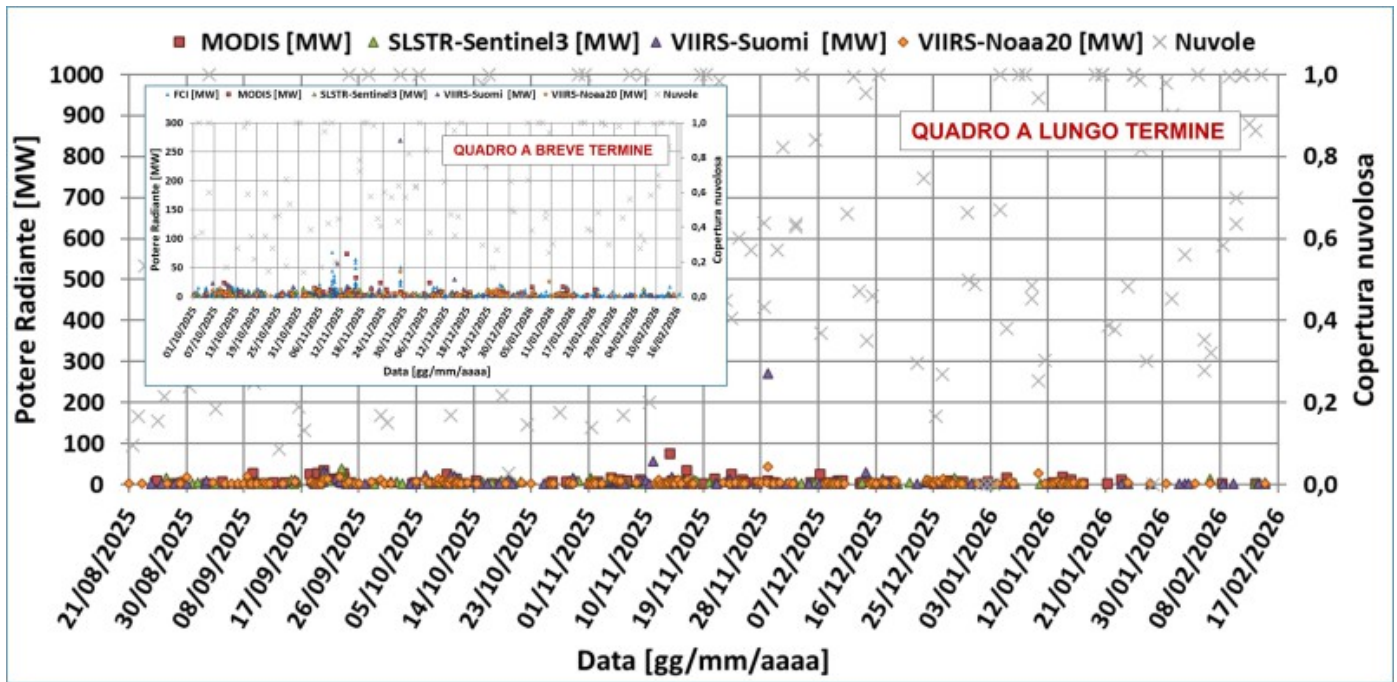
Fig. 7.1 Potere radiante calcolato da dati MODIS (quadrato rosso), SENTINEL-3 SLSTR (triangolo verde), VIIRS (triangolo viola e rombo giallo) e MTG-FCI (triangolo blu) dal 21 agosto 2025 al 17 febbraio 2026.
