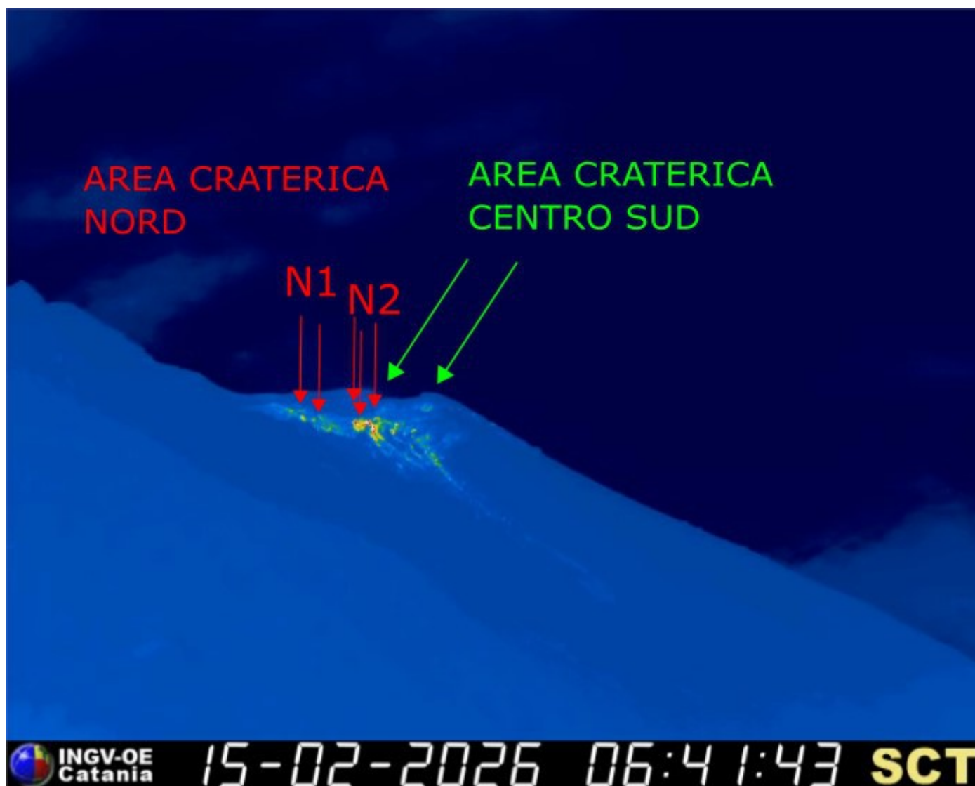
Fig. 3.1 La terrazza craterica vista dalla telecamera termica posta a quota 190 m con la delimitazione delle aree crateriche Area Centro-Sud e Area Nord. Le frecce indicano le ubicazioni delle bocche attive.
